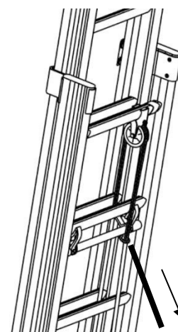
Abbildung 14: Seilführung
